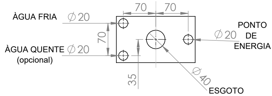
Esquema de instalação (Sob acento)
